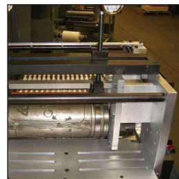
Inner Sideframe
